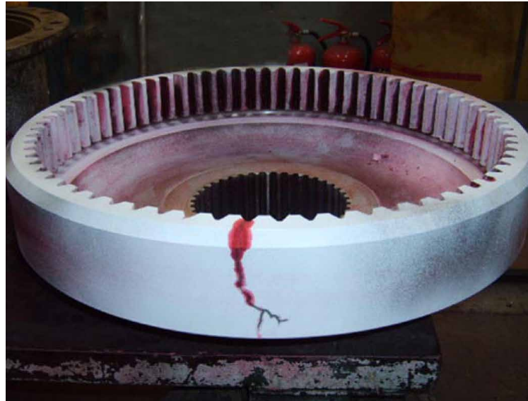
Inspecciones No Destructivas, esta foto muestra una grieta en una corona de reductor, cuya reparación se efectúa según muestra original
