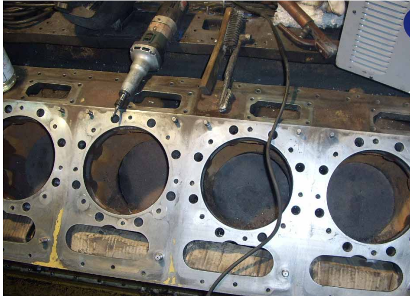
Reparación de block de Motor en Pasada de Agua de Enfriamiento. Sistema con Arco Manual (Material Fierro Fundido)
